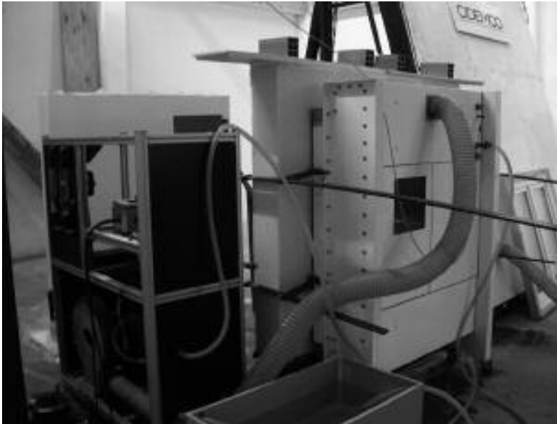
Fotografía n°1: Equipamiento de ensayo para el procedimiento CIDEMCO CO-115
